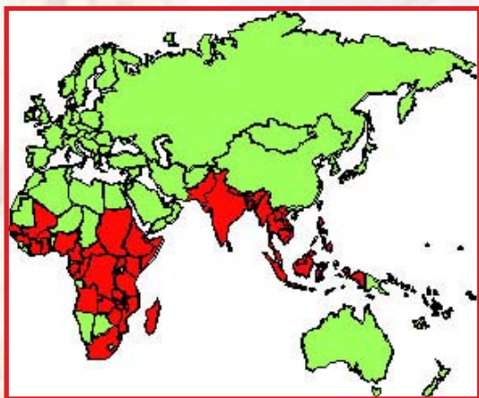
Фиг. 12. Географско разпространение на чикунгуња
